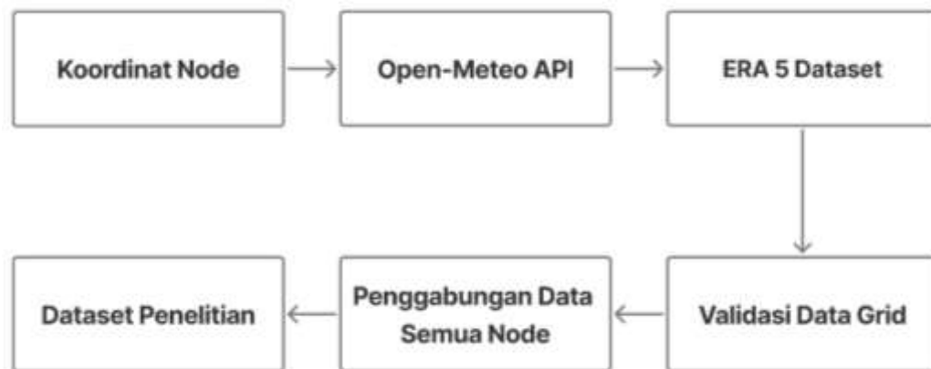
Gambar 3.2 Diagram Proses Pengambilan Data ERA5 melalui Open-Meteo API
